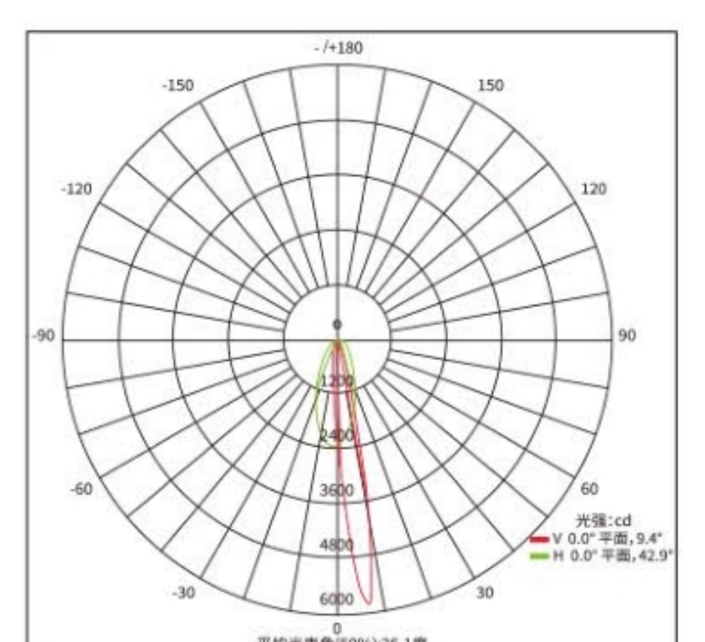
配光曲线
